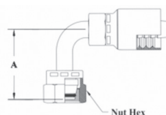
DIN HEAVY 24° SEAT- FEMALE SWIVEL 90° BEND
