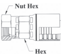
DIN Heavy 24° Seat Female Swivel
