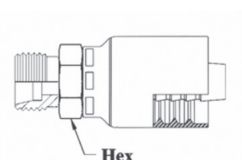
DIN HEAVY 24° SEAT- MALE SOLID
